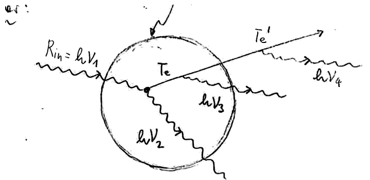
Slika 30: Energijska bilanca kerme v volumnu V . Vpadni foton R_{in} = h\nu_1 interagira v volumnu; nastali nabiti delci (npr. elektron s kinetično energijo T_e ) in sipani/sekundarni fotoni ( h\nu_2, h\nu_3, h\nu_4, T'_e ) zapustijo volumen.
