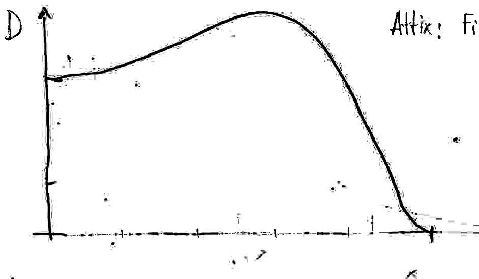
Slika 43: Attix, slika 8.14 (a): Tipična porazdelitev doze D(x) za elektrone. Doza sprva narašča (kopičenje sekundarnih elektronov), doseže maksimum in nato upade; globina je izražena v enotah masne debeline x/\rho .
