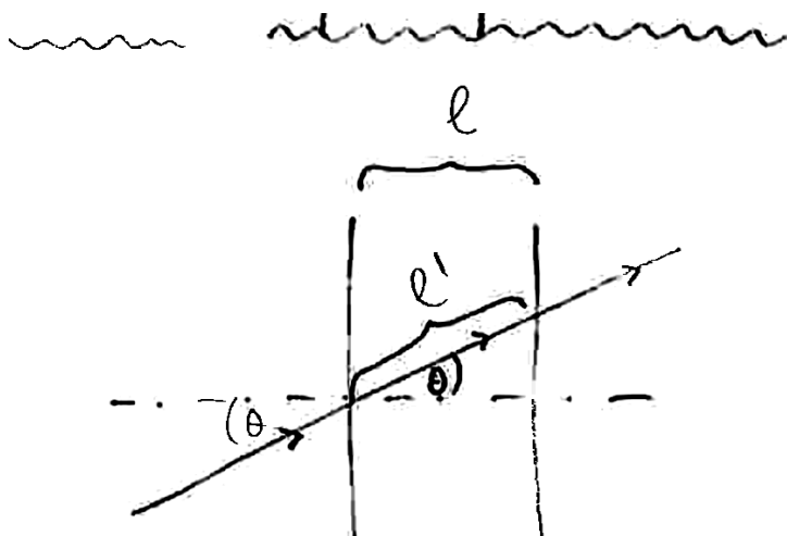
Slika 38: Vpad pod kotom \theta na plast debeline l . Dolžina poti skozi plast je l' = l / \cos \theta .
