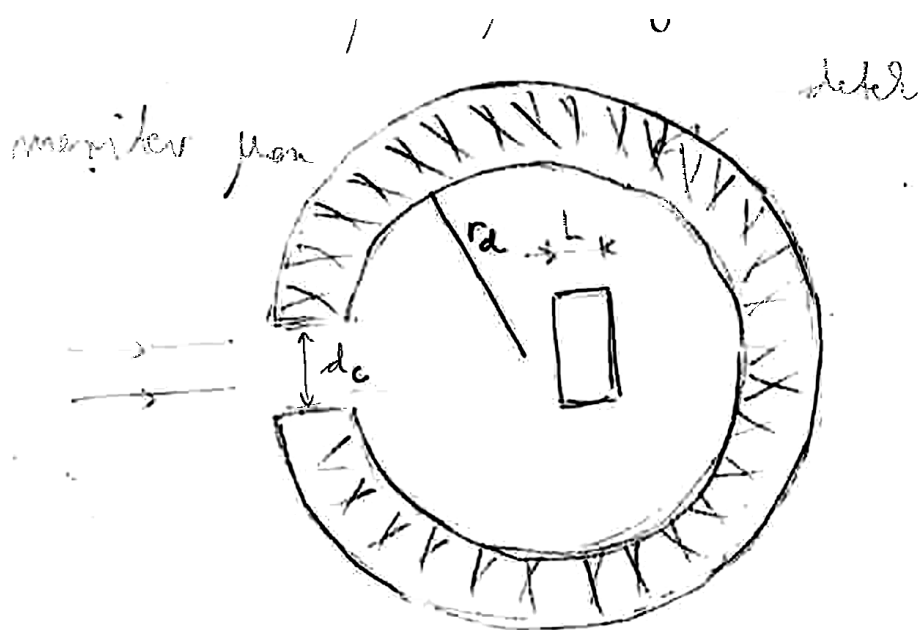
Slika 29: Idealna geometrija za meritev \mu_{en} . Detektor je obdan s snovjo, radij detektorja r_d pa je velik v primerjavi z debelino attenuatorja d_c ( r_d \gg d_c ), zato vsi sipani fotoni dosežejo detektor.
