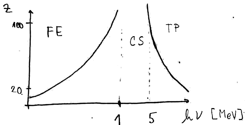
Slika 15: Attix, slika 7.1: Diagram dominantnih področij interakcije fotonov (FE, CS, TP) v odvisnosti od energije fotona ( h\nu ) in vrstnega števila absorbenta ( Z ). Črte predstavljajo meje, kjer sta verjetnosti za dva sosednja procesa enaki.
