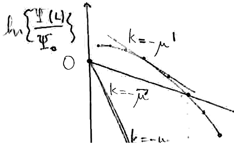
Slika 28: Attix, slika 3.4 (b): \ln(\Psi(L)/\Psi_0) v odvisnosti od globine L za točkast izvor v vodi ( h\nu = 0.279 \text{ MeV} ). Pri majhnih globinah je zaradi faktorja kopičenja naklon drugačen; asimptotični naklon ustreza \bar{\mu}' , začetni pa -\mu .
