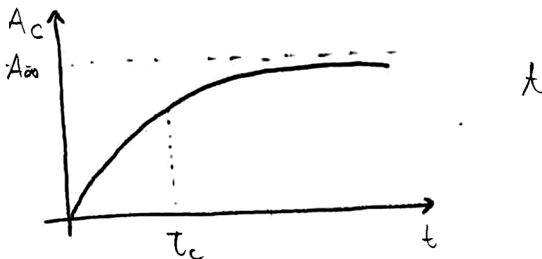
Slika 9: Naraščanje aktivnosti A_C(t) med aktivacijo s konstantnim fluksom projektilov. Aktivnost se asimptotično približuje nasičeni vrednosti A_\infty = N_{B,0}\Phi\sigma s časovno konstanto \tau_C = 1/\lambda_C .
