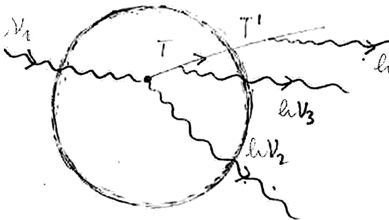
Slika 33: Bilanca deponirane energije v volumnu V . Vpadni foton h\nu_1 se sipa ( h\nu_2 ), elektron s kinetično energijo T del energije izgubi z zavornim sevanjem ( h\nu_3 ) in izstopi s preostalo energijo T' ; zunaj volumna izseva še foton h\nu_4 .
