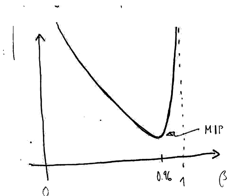
Slika 34: Masna ustavljalna moč |dT/\rho dx| v odvisnosti od relativne hitrosti \beta . Pri \beta \approx 0.96 ima minimum (minimalno ionizirajoči delci), pri \beta \rightarrow 1 pa zaradi relativističnega dviga strmo narašča.
