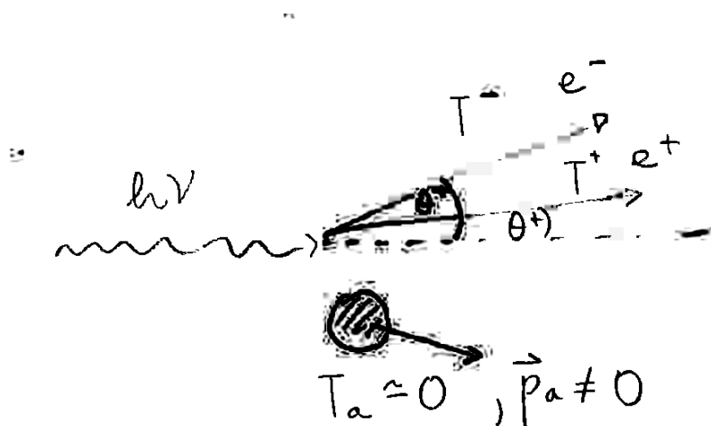
Slika 22: Tvorba para v električnem polju jedra. Foton h\nu ustvari elektron in pozitron, jedro pa prevzame gibalno količino ( T_a \approx 0 , p_a \neq 0 ).
