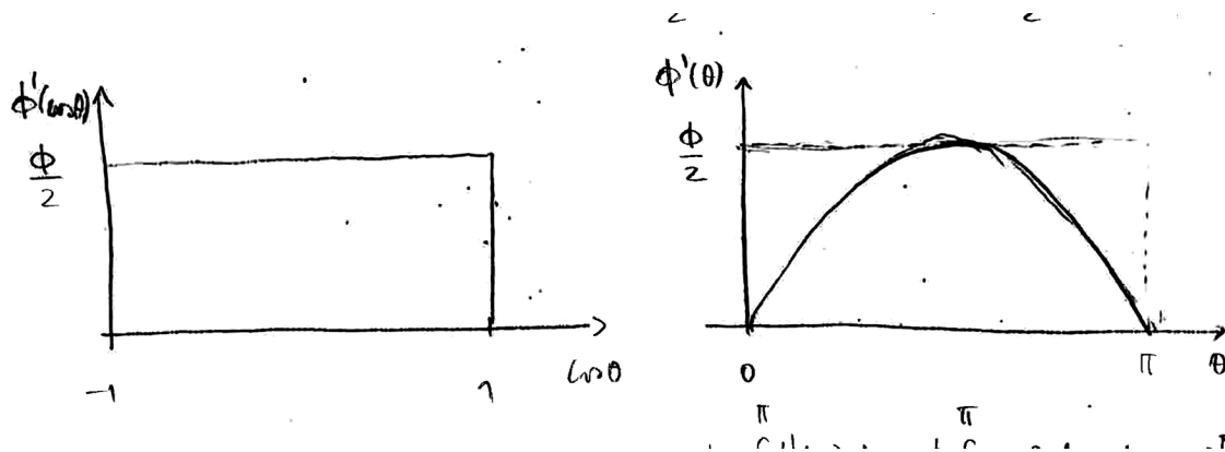
Slika 13: Primerjava porazdelitve gostote toka za izotropno sevalno polje. Levo: porazdelitev po \cos\theta je konstantna in znaša \phi/2 . Desno: porazdelitev po \theta sledi funkciji \phi'(\theta) = \frac{\phi}{2} \sin\theta . Ploščina pod obema krivuljama je enaka in predstavlja celotno gostoto toka \phi .
