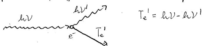
Slika 4: Skica Comptonovega sipanja. Vpadni foton h\nu se siplje na elektronu v smer h\nu' in mu preda del svoje energije; kinetična energija Comptonovega elektrona je T_e' = h\nu - h\nu' .
