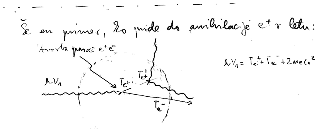
Slika 32: Tvorba para z anihilacijo v letu. Foton h\nu_1 ustvari par e^-e^+ ; pozitron anihilira, še preden se popolnoma ustavi, zato nastala fotona odneseta dodatno kinetično energijo T'_{e^+} .
