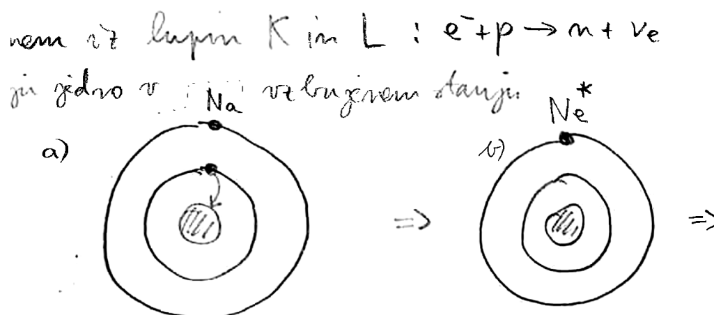
Slika 7: Zajetje elektrona (EC). (a) Jedro zajame elektron iz notranje lupine (najpogosteje K ali L) in odda nevtrino; nastane vzbujeno hčerinsko jedro. (b) Vzbujeno jedro ^{22}\text{Ne}^* se relaksira z izsevanjem žarka gama.
