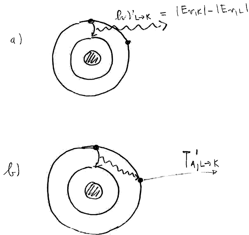
Slika 3: Relaksacija atoma z vrzeljo v lupini K. (a) Vrzal se zapolni z elektronom iz višje lupine L, razlika energij pa se izseva kot karakteristični žarek X z energijo h\nu'_{L \rightarrow K} = |E_{v,K}| - |E_{v,L}| . (b) Energija se prenese na elektron v višji lupini, ki ga izbije kot Augerjev elektron s kinetično energijo T'_{A,L \rightarrow K} .
