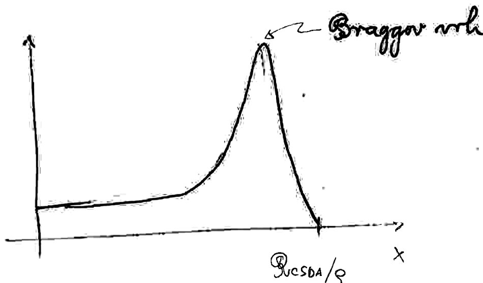
Slika 41: Braggova krivulja: lokalna doza D(x) težkih nabitih delcev v odvisnosti od globine. Pred koncem dosega R_{CSDA}/\rho doza izrazito naraste (Braggov vrh), nato strmo pade na nič.
