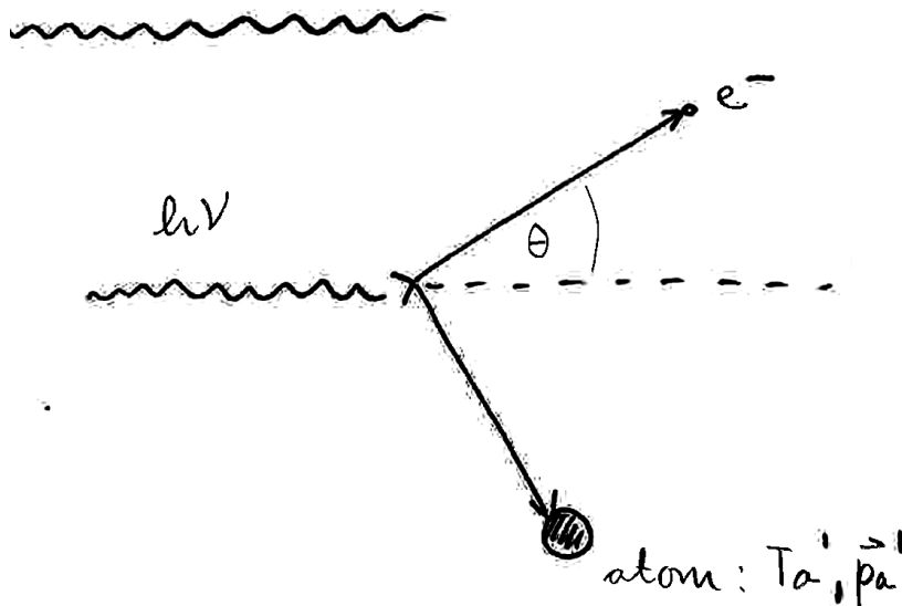
Slika 20: Kinematika fotoefekta. Foton h\nu izbije fotoelektron pod kotom \theta ; preostanek atoma (ion) prevzame gibalno količino in kinetično energijo T_a .
