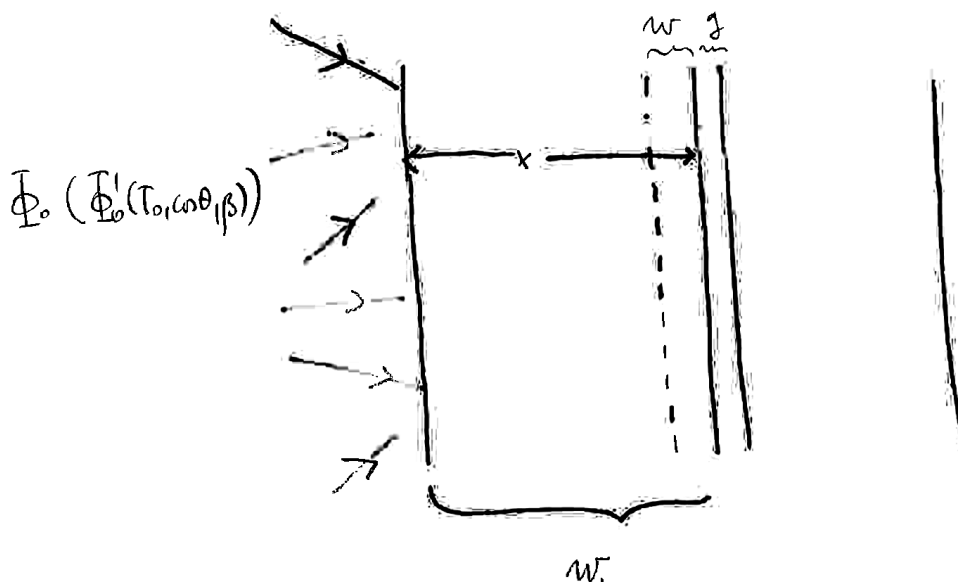
Slika 45: Shema votlinske teorije. Votlina (plin) g je obdana s stenama w in w_L ; na votlino vpadla fluenca nabitih delcev \Phi_0 s spektrom \Phi'_0(T_0) .
