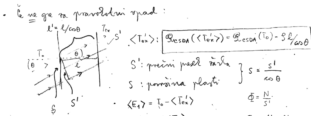
Slika 39: Poševni vpad delcev na plast. Prečni presek žarka je S' , površina plasti pa S = S'/\cos\theta ; izstopna energija je \langle T'_{ex} \rangle .
