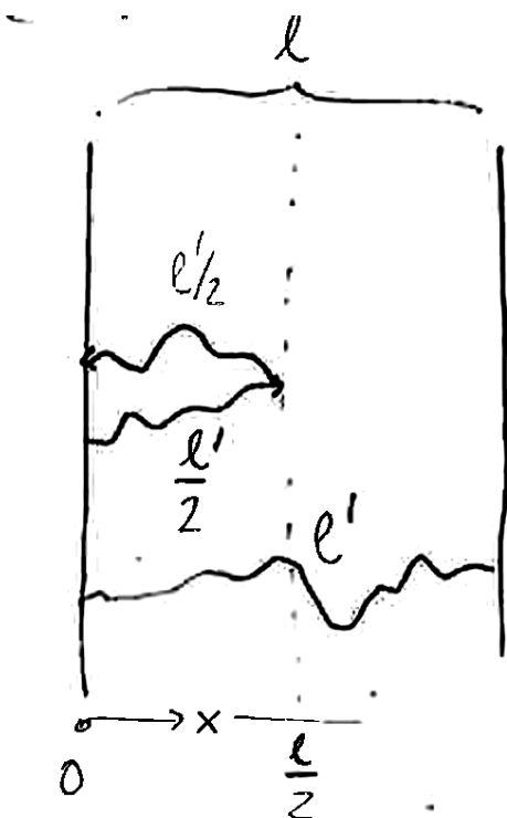
Slika 42: Vpliv povratnega sipanja v tanki plasti. Elektron se v povprečju povratno siplje na globini x \approx l/2 ; skupna prepotovana dolžina v plasti ostane l'/2 + l'/2 = l' .
