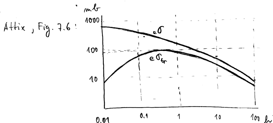
Slika 19: Attix, slika 7.6: Totalni presek za Comptonovo sipanje {}_e\sigma in presek za prenos energije {}_e\sigma_{tr} v odvisnosti od energije vpadnega fotona h\nu .
