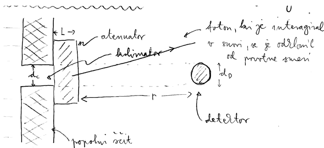
Slika 25: Geometrija ozkega snopa. Kolimatorja oblikujeta ozek snop, attenuator debeline L pa je daleč od detektorja ( r \gg d_C, d_D ), zato sipani fotoni zgrešijo detektor.
