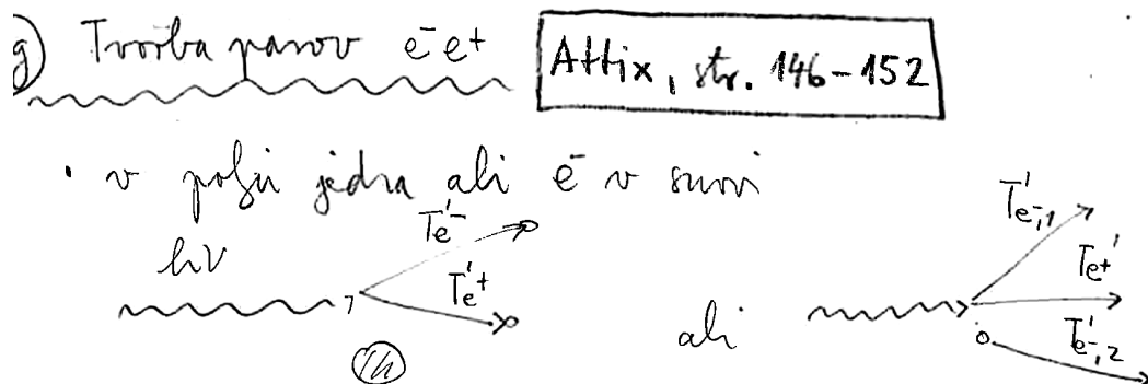
Slika 5: Tvorba para elektron-pozitron. Levo: tvorba v polju atomskega jedra, kjer jedro prevzame odvečno gibalno količino ( T_a \approx 0 , p_a \neq 0 ). Desno: tvorba tripleta v polju atomskega elektrona, kjer nastanejo trije delci ( e_1^-, e_2^-, e^+ ).
