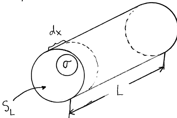
Slika 17: Geometrija za definicijo sipalnega preseka. Vsako sipalno središče (kroglice) ima presek \sigma ; tarča ima prečni presek S_L in dolžino L . Verjetnost interakcije v tankem sloju dx je sorazmerna z n_L \sigma dx .
