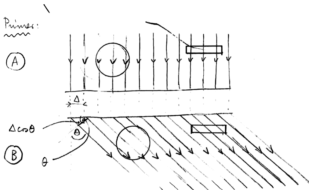
Slika 14: Vpliv geometrije polja na meritev fluence. (A) Homogeno polje s pravokotnim vpadom (razdalja med sosednjima žarkoma \Delta ). (B) Homogeno polje s poševnim vpadom pod kotom \theta (razdalja med žarkoma \Delta \cos \theta ). Razmerja izmerjenih fluenc s kroglo in diskom se med poljema A in B razlikujejo.
