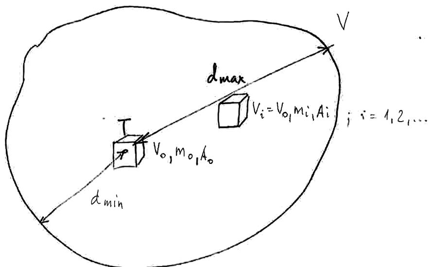
Slika 44: Geometrija recipročnega izreka. Volumen V je homogeno zapolnjen s sevalci; V_0 je referenčni volumen, V_i poljubni volumen, d_{min} in d_{max} pa najmanjša in največja razdalja do roba snovi.
