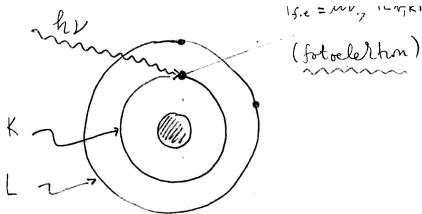
Slika 2: Fotoelektrični pojav. Vpadni foton h\nu izbije elektron iz notranje lupine (K ali L), pri čemer v atomu ostane prazno mesto (vrzel). Kinetična energija fotoelektrona je T_{f,e} = h\nu - |E_{v,K}| .
