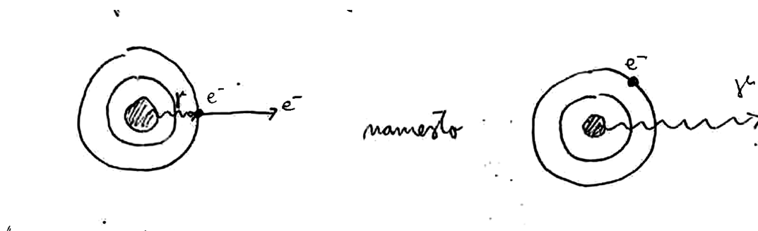
Slika 6: Notranja konverzija. Levo: vzbujeno jedro preda energijo elektronu iz elektronske ovojnice in ga izbije (notranja konverzija). Desno: alternativno se jedro relaksira z izsevanjem žarka gama.
