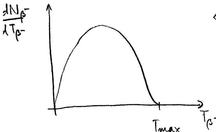
Slika 1: Zvezni energijski spekter delcev \beta^- pri razpadu {}^{32}\text{P} . Porazdelitev dN_{\beta^-}/dT_{\beta^-} sega od nič do maksimalne energije T_{\max} = 1.71 \text{ MeV} .
