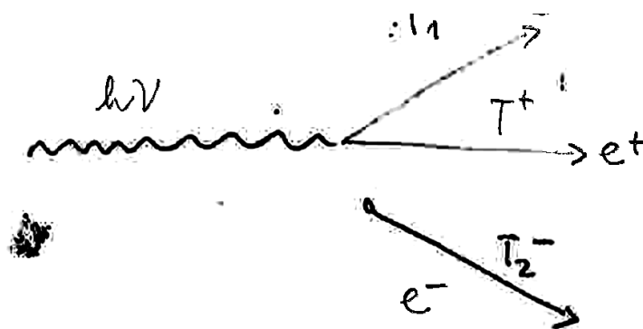
Slika 23: Tvorba para v polju atomskega elektrona (tvorba tripleta). Končni produkti so trije delci: pozitron ter dva elektrona.
