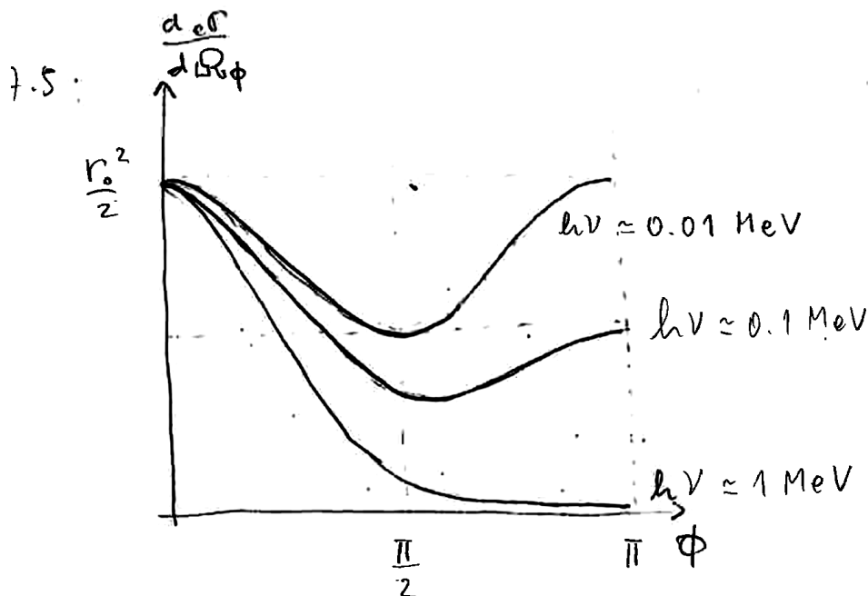
Slika 18: Attix, slika 7.5: Diferencialni presek Kleina-Nishine v odvisnosti od sipalnega kota fotona \phi za različne energije vpadnega fotona h\nu . Pri nizkih energijah (npr. 0.01 MeV) je porazdelitev skoraj simetrična (podobna Thompsonovi), medtem ko pri višjih energijah postane močno usmerjena naprej.
