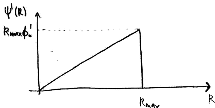
Slika 12: Ustrezni energijski spekter gostote energijskega toka \psi'(R) = R \phi'(R) , ki linearno narašča do vrednosti R_{\max} \phi'_0 pri R = R_{\max} .
