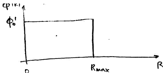
Slika 11: Ravni energijski spekter gostote toka delcev: \phi'(R) = \phi'_0 za 0 \leq R \leq R_{max} in nič sicer.
