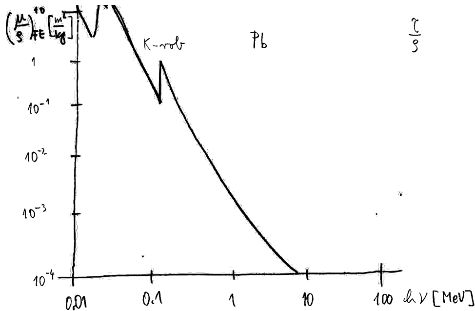
Slika 21: Attix, slika 7.13: Masni koeficient fotoefekta (\mu/\rho)_{\text{FE}} za svinec (Pb) v odvisnosti od energije fotona. Opazen je izrazit K-rob pri vezavni energiji K-lupine.
