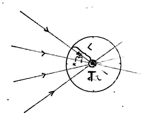
Slika 24: Idealizirana postavitev z majhno detektorsko kroglico s presekom S okoli točke T . Vsak žarek, ki leti proti detektorju, prepotuje skozi absorbent pot dolžine L .
